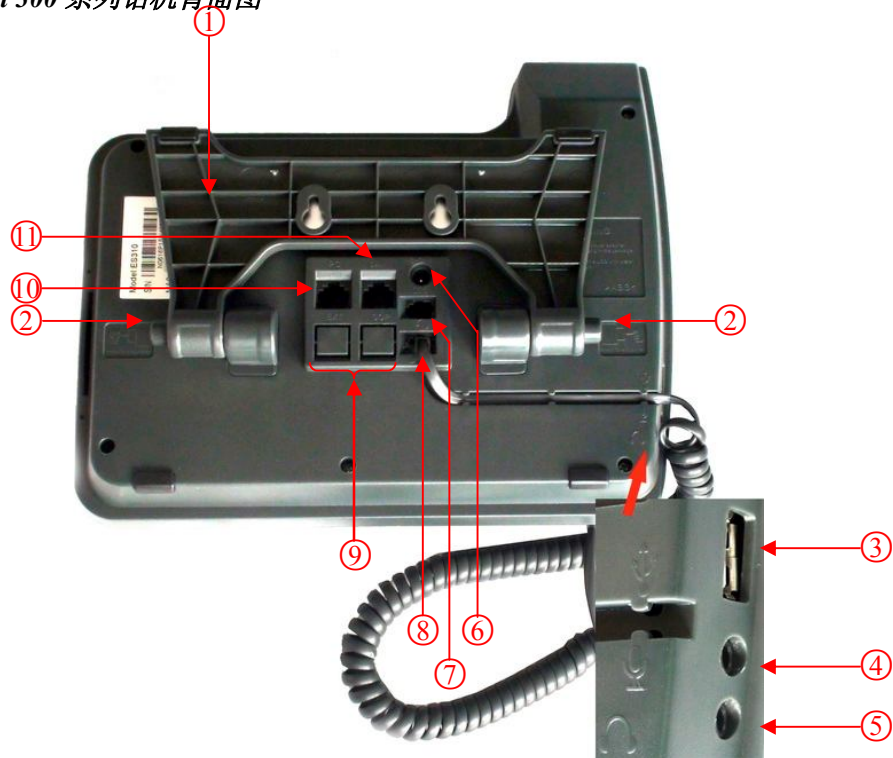
图 3.2 SayHi 300 系列话机背面图
