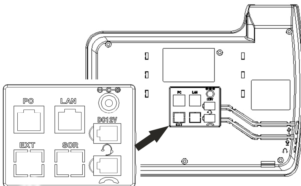
图 2.1 SayHi 300 系列话机背部连接接口
